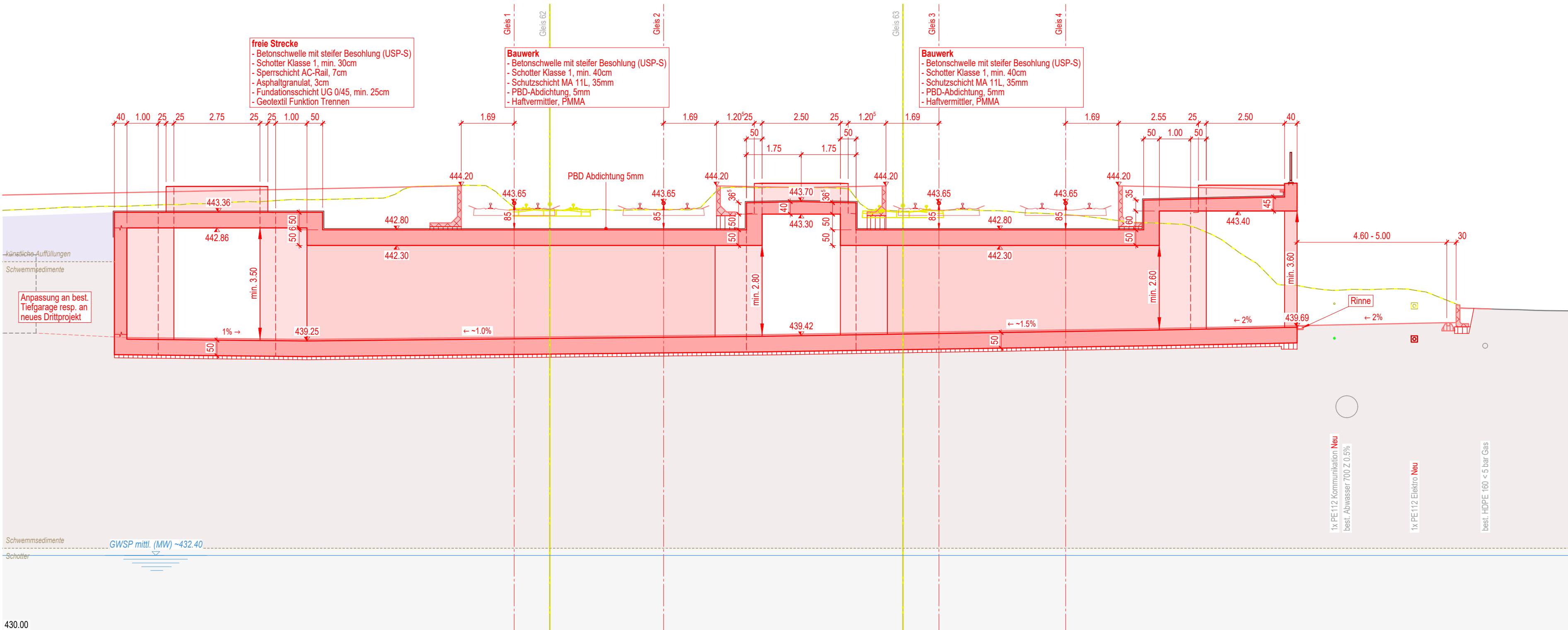
Schnitt 1-1, 1:100
